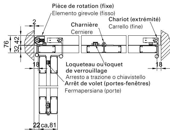
2 Vantaux, schéma 0L -2R | 2 ante, schema 0L-2R
