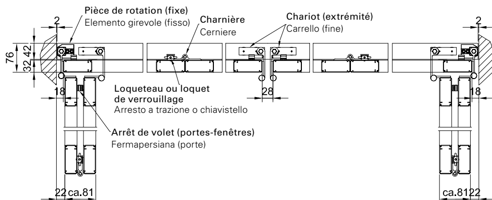
4 Vantaux, schéma 0L -2R | 4 ante, schema 0L-2R
