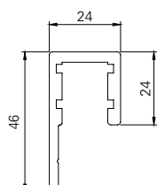
Profil de guidage inférieur Profilo di guida inferiore
