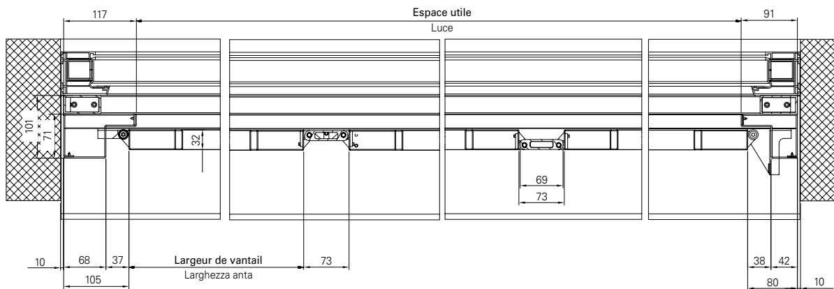
Coupe horizontale
