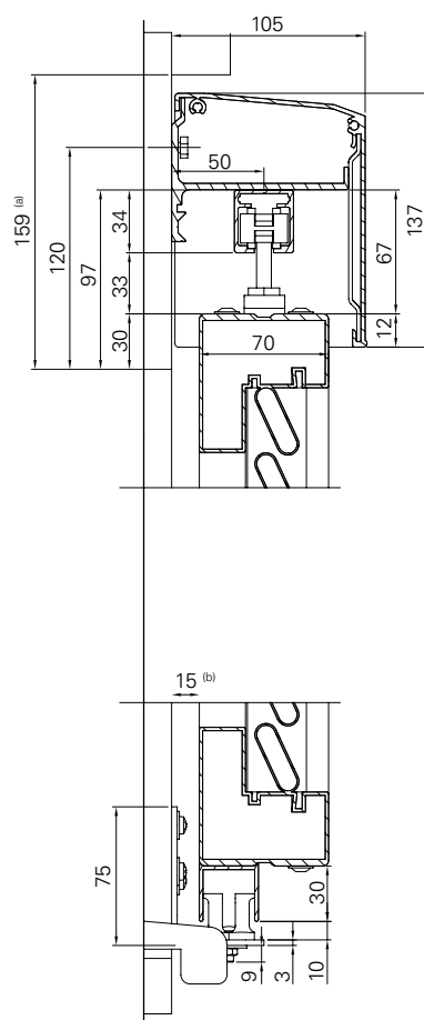
Système A105 | ECO 60 | BT 70 | Type A Sistema A105 | ECO 60 | BT 70 | Tipo A
