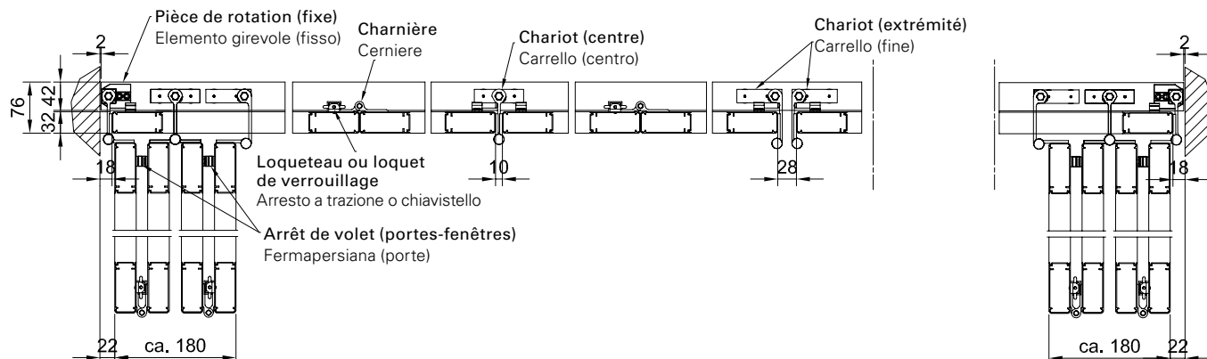
8 Vantaux, schéma 0L -4R | 8 ante, schema 0L-4R
