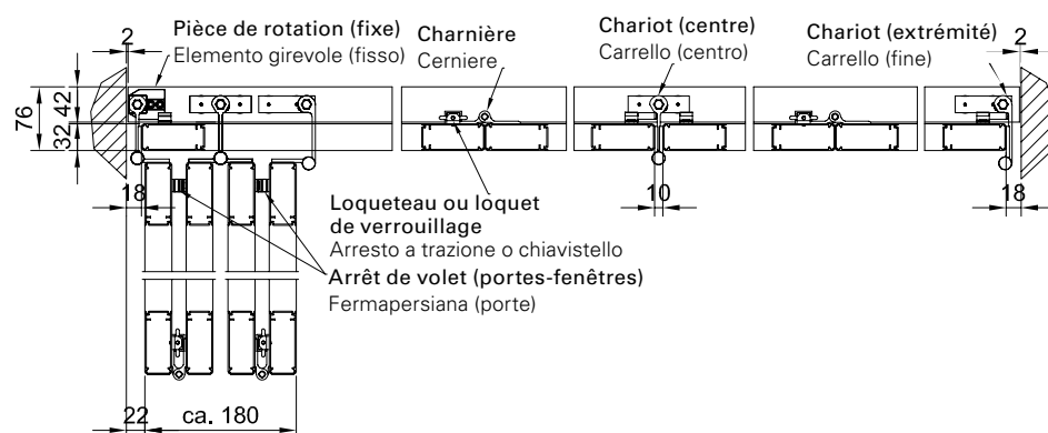
4 Vantaux, schéma 0L -4R | 4 ante, schema 0L-4R
