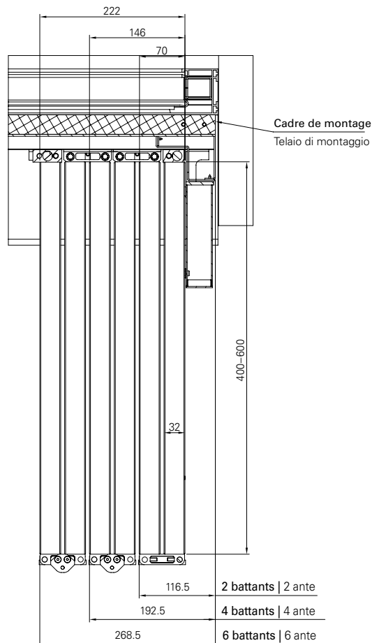
Coupe du système (dimension du paquet)
