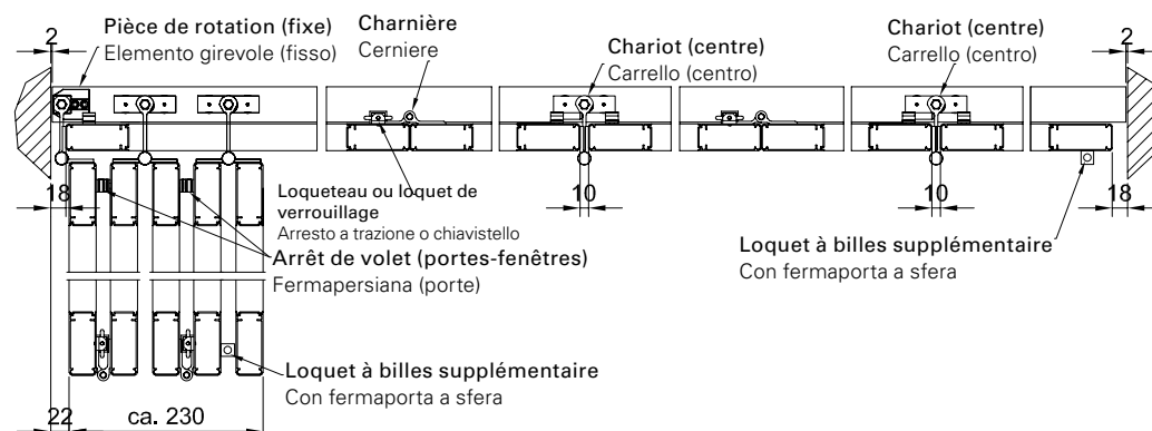
5 Vantaux, schéma 0L -5R | 5 ante, schema 0L-5R
