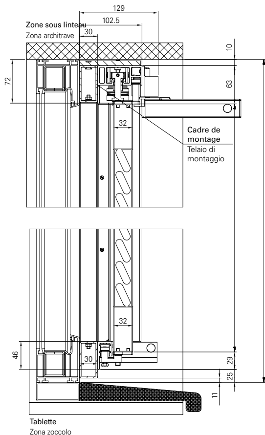
Coupe verticale
