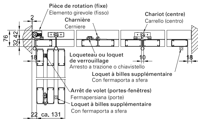
3 Vantaux, schéma 0L -3R | 3 ante, schema 0L-3R
