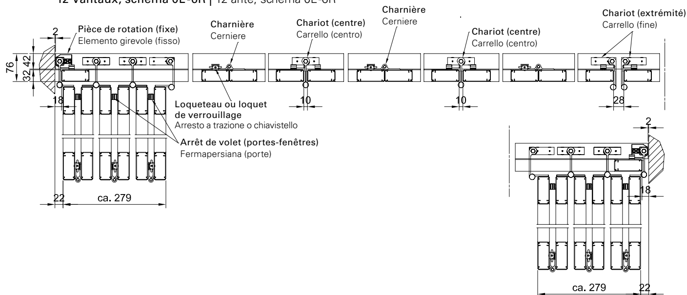
12 Vantaux, schéma 0L -6R | 12 ante, schema 0L-6R
