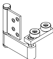
Chariot Carrello di guida
